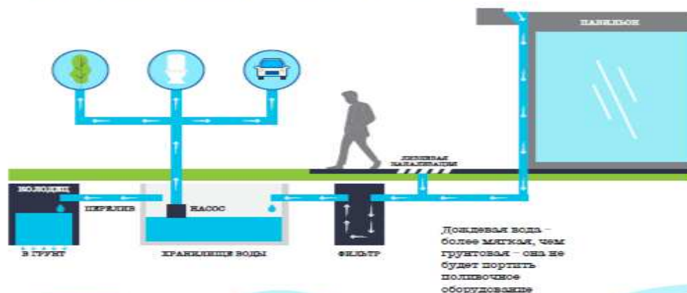
СХЕМА ПРОЕКТНОГО РЕШЕНИЯ ПО СБОРУ И УТИЛИЗАЦИИ ВОДЫ
